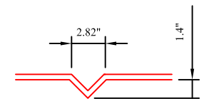
BAFFLE RIB DETAIL SCALE: N.T.S.
